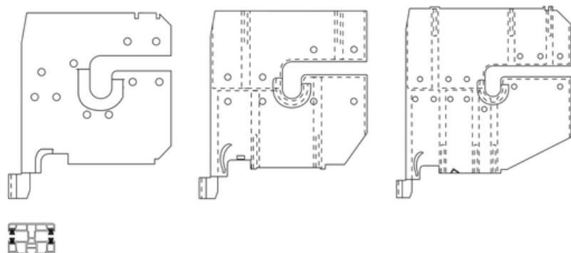
RKM 101 OSZTÓPOFA 135 MM EGYLEFUTÓS VÁLTOZAT - kétoldalon kefézett PVC lefutósínhez
