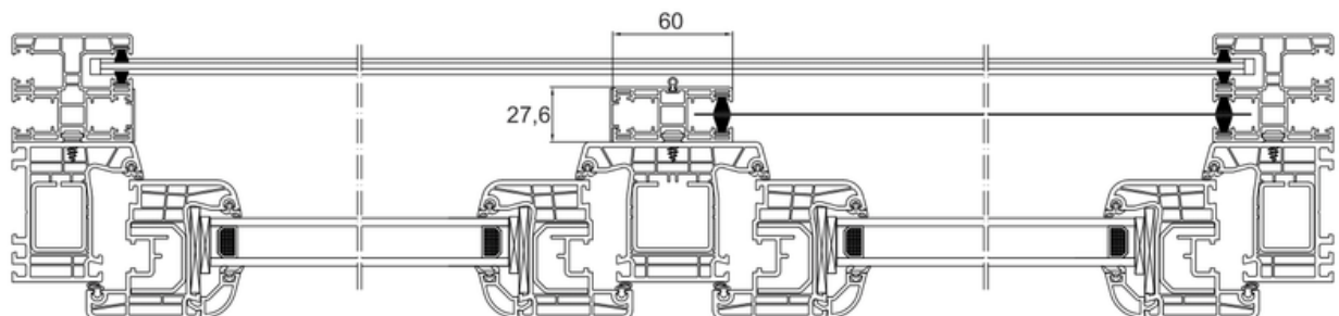
Szúnyogháló lefutó alkalmazása: (NPD-070, NPR-030)
