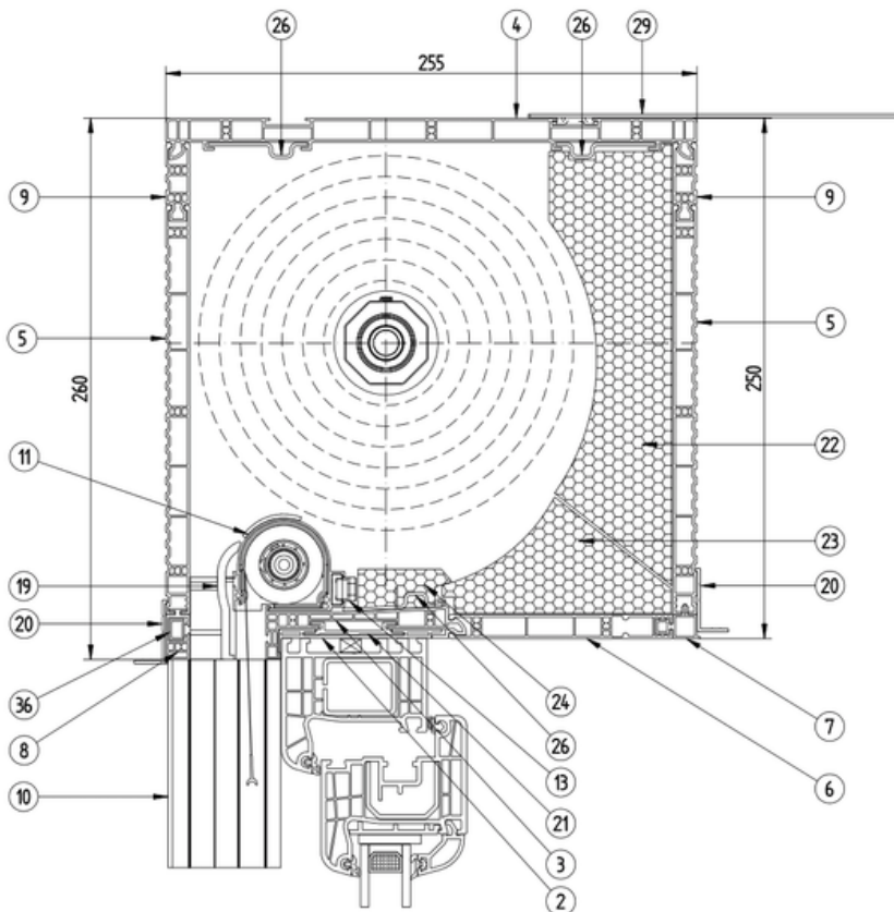
250mm-es, rovarhálós tok szerelőfedelének elhelyezkedési lehetőségei
