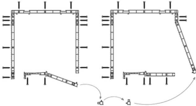
250mm-es, rovarhálós tok szerelőfedelének elhelyezkedési lehetőségei
